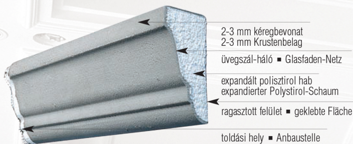
Ablakkerettel keretezve
